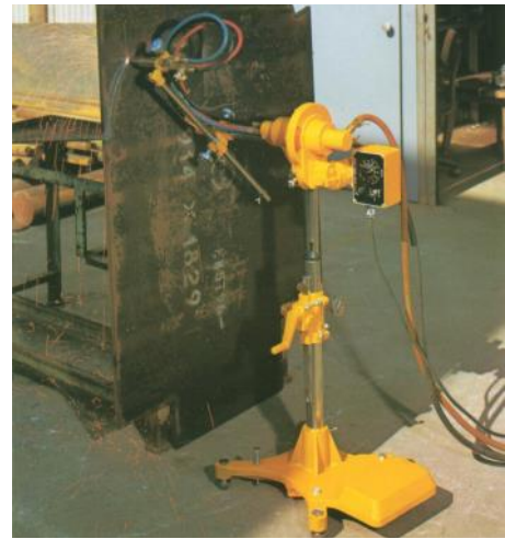
Verticaal snijden
