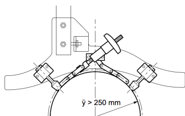
Зажимное приспособление для труб малых диаметров
