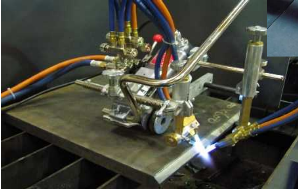
端面倣い開先切断機 「IK-93 EDGE-CUT」
