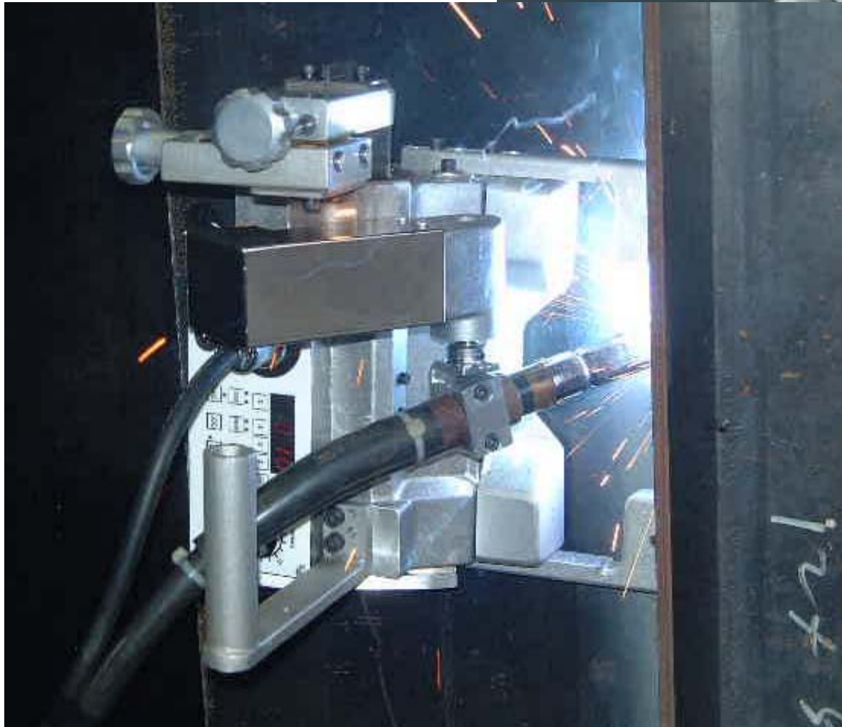
溶接機 ウェルハンディ マルチ シリーズ
